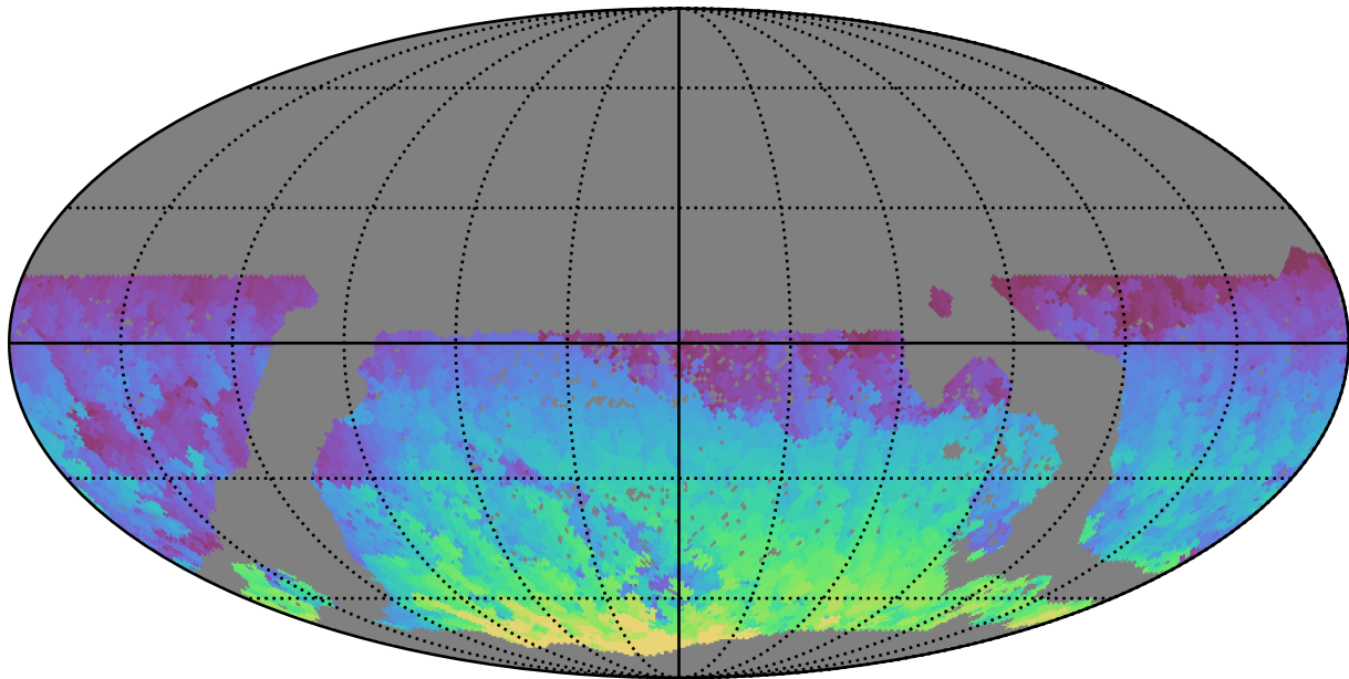
mw_roll_all_v3.3_10yrs WFD i band: Max HA
