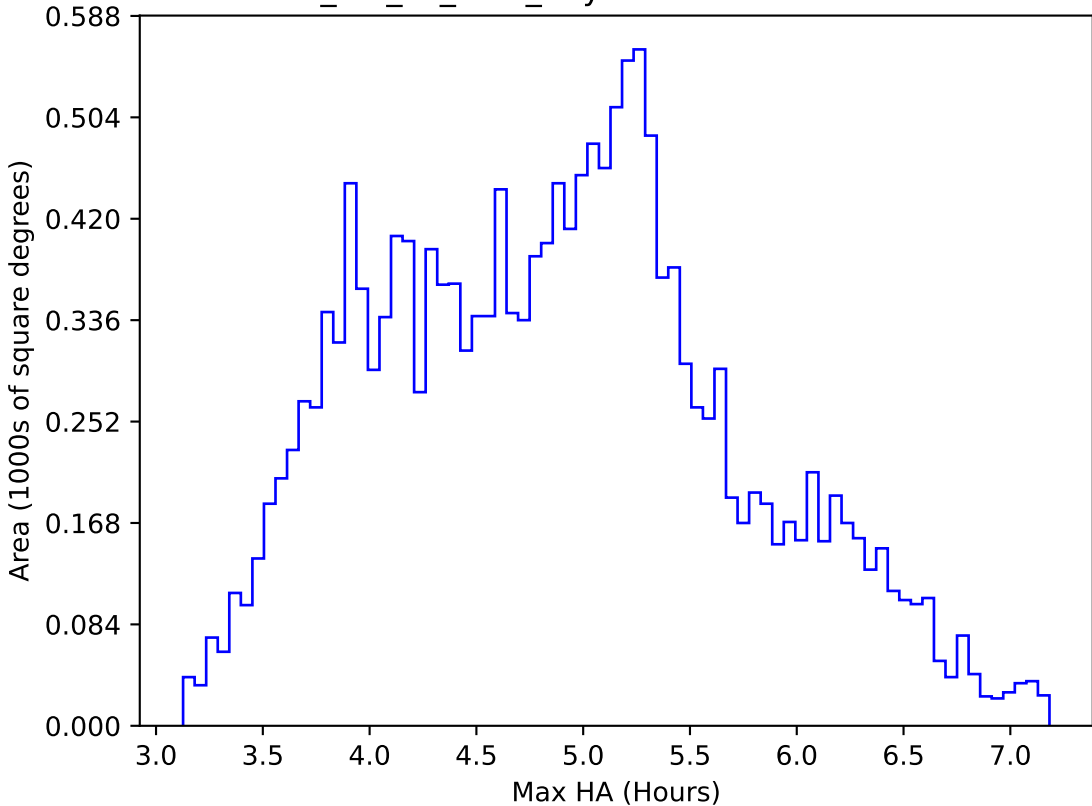
mw_roll_all_v3.3_10yrs WFD i band: Max HA
