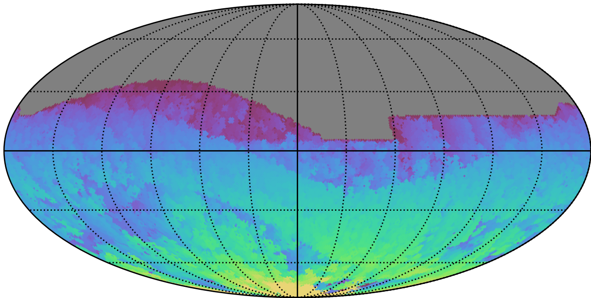
mw_roll_all_v3.3_10yrs All sky z band: Max HA
