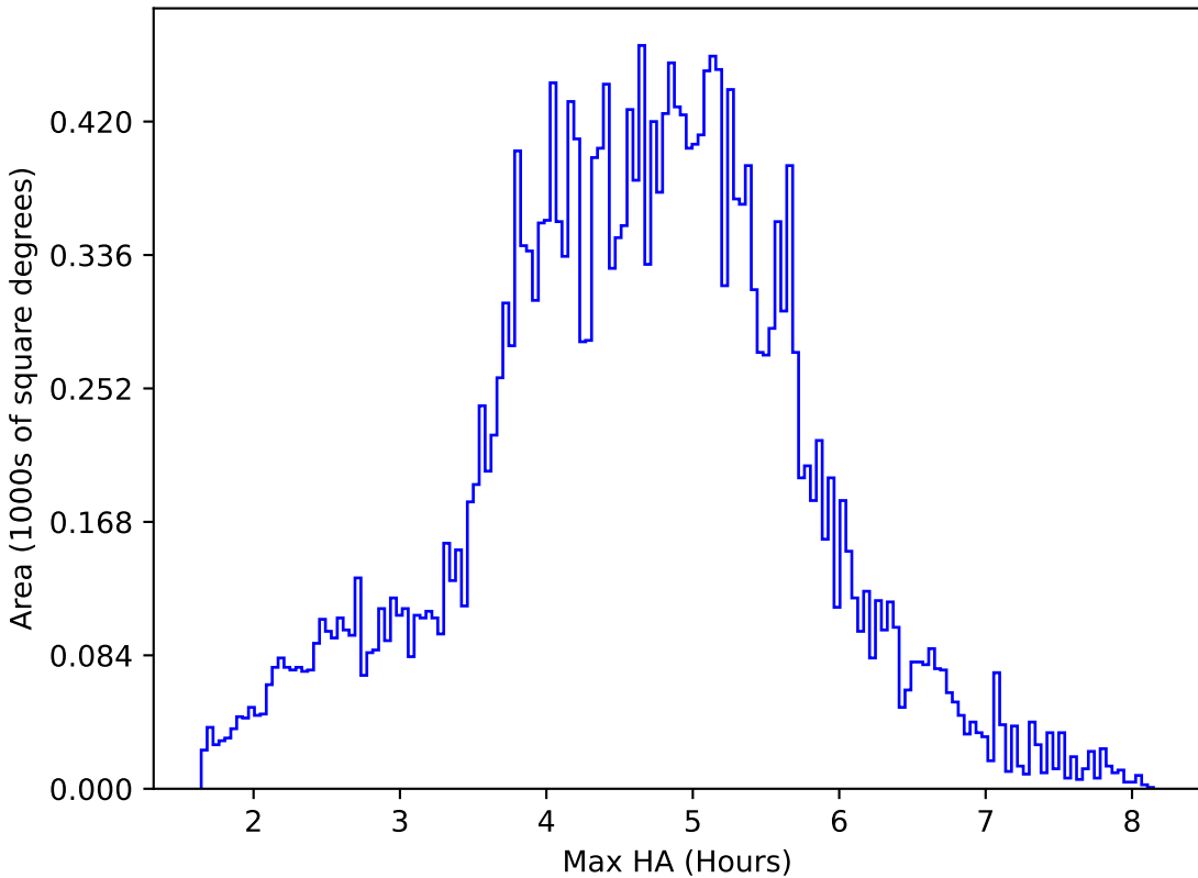
mw_roll_all_v3.3_10yrs All sky z band: Max HA
