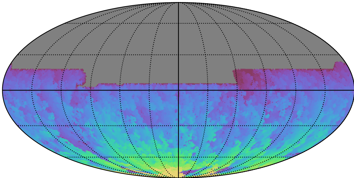
mw_roll_all_v3.3_10yrs All sky y band: Max HA
