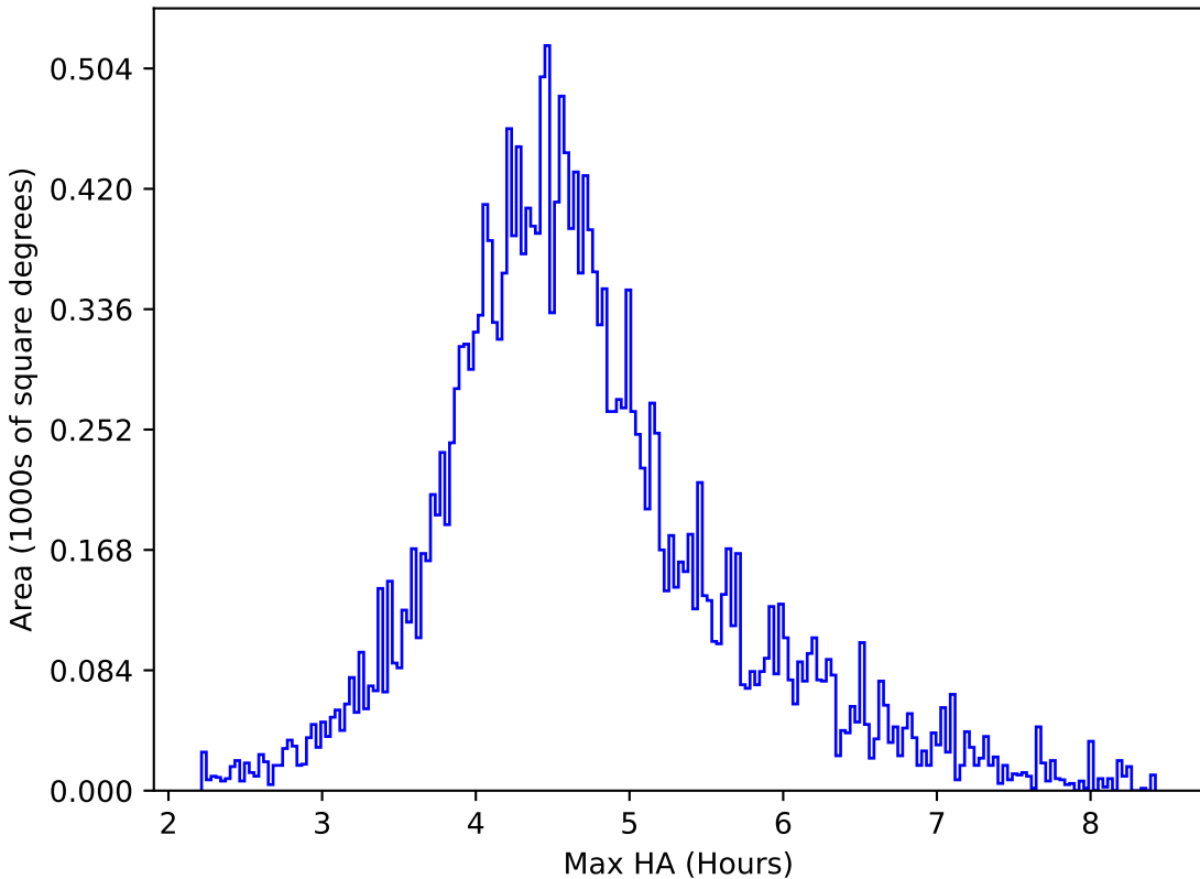
mw_roll_all_v3.3_10yrs All sky y band: Max HA
