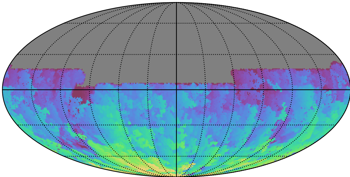
mw_roll_all_v3.3_10yrs All sky u band: Max HA
