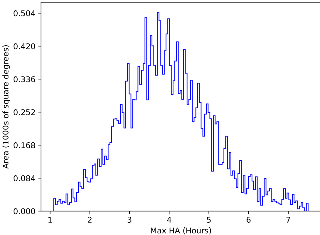
mw_roll_all_v3.3_10yrs All sky u band: Max HA
