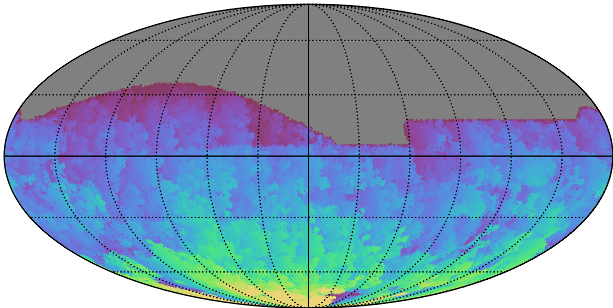
mw_roll_all_v3.3_10yrs All sky r band: Max HA
