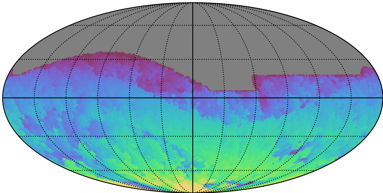
mw_roll_all_v3.3_10yrs All sky i band: Max HA
