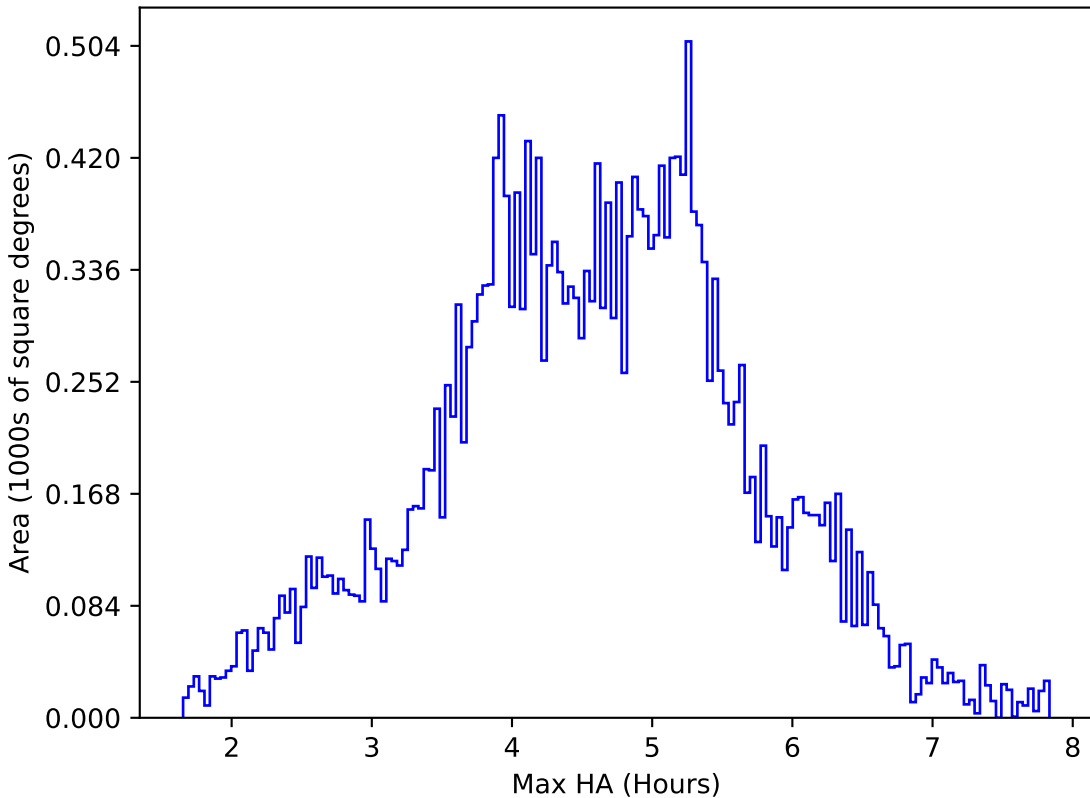
mw_roll_all_v3.3_10yrs All sky i band: Max HA
