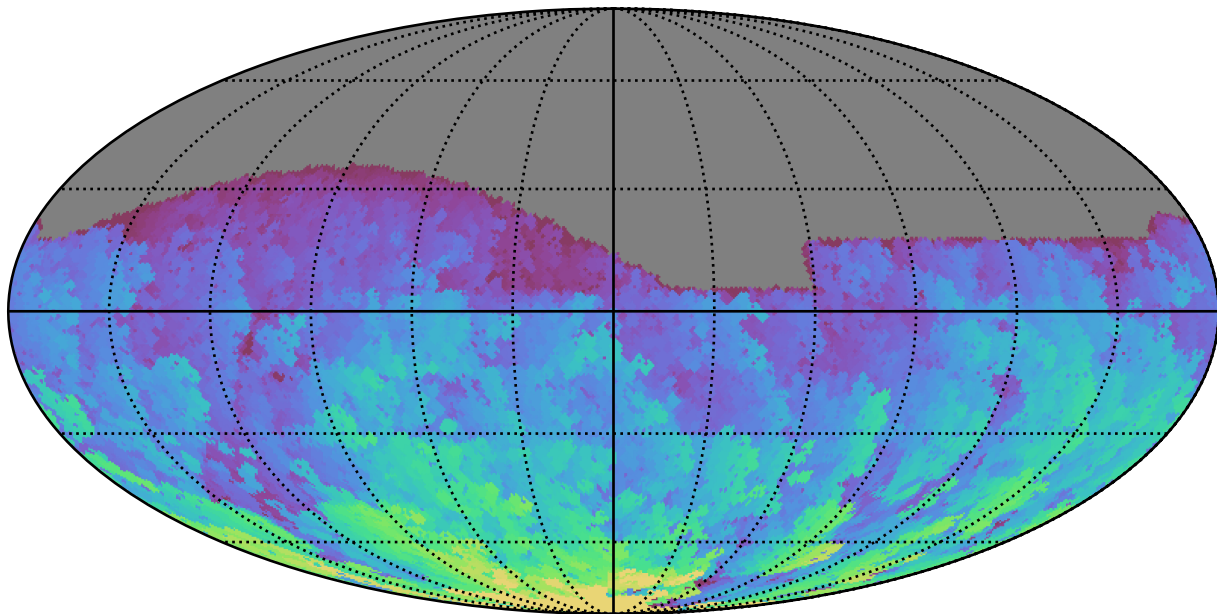
mw_roll_all_v3.3_10yrs All sky g band: Max HA
