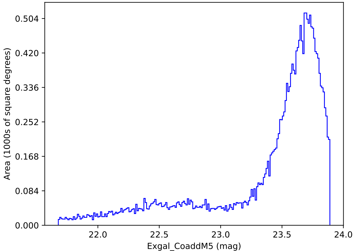
mw_roll_all_v3.3_10yrs Yr 1 y band: Exgal_CoaddM5
