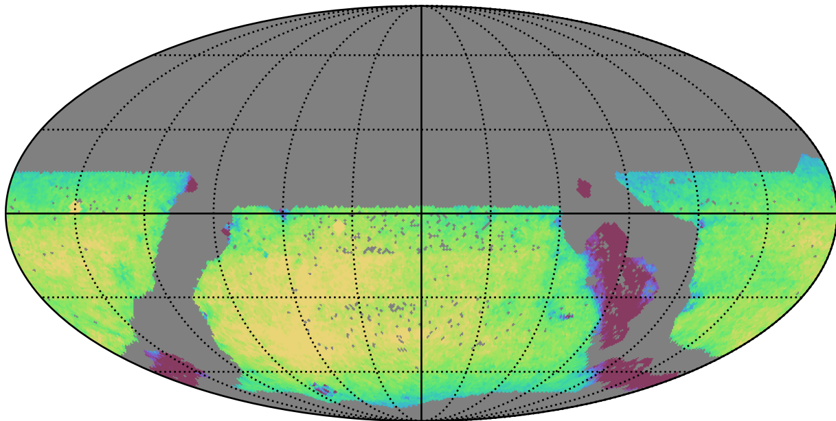
mw_roll_all_v3.3_10yrs WFD y band: Exgal_CoaddM5
