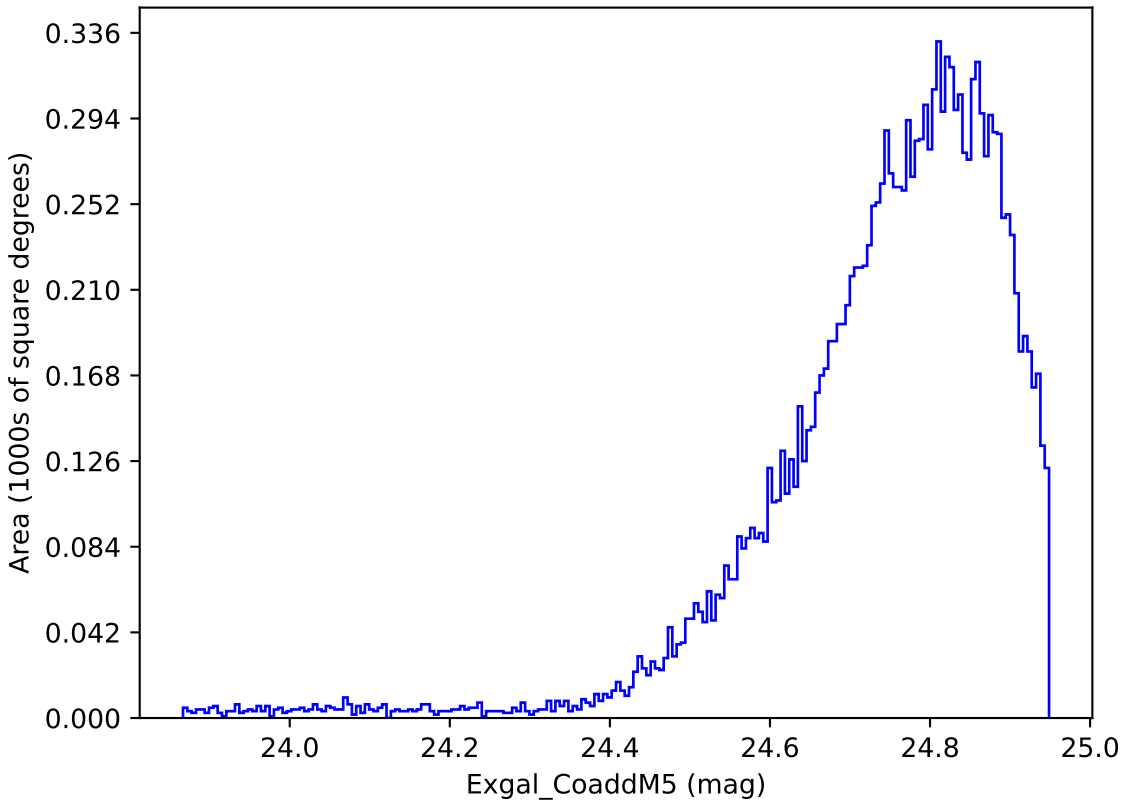
mw_roll_all_v3.3_10yrs WFD y band: Exgal_CoaddM5
