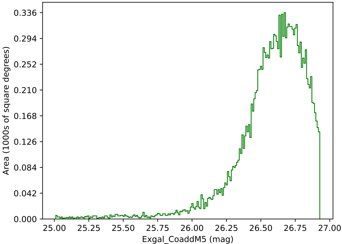
mw_roll_all_v3.3_10yrs WFD g band: Exgal_CoaddM5
