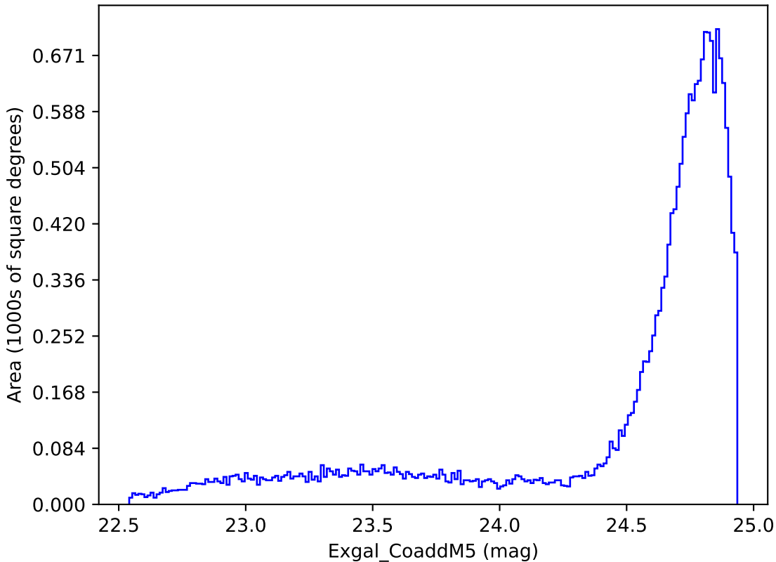
mw_roll_all_v3.3_10yrs All sky y band: Exgal_CoaddM5
