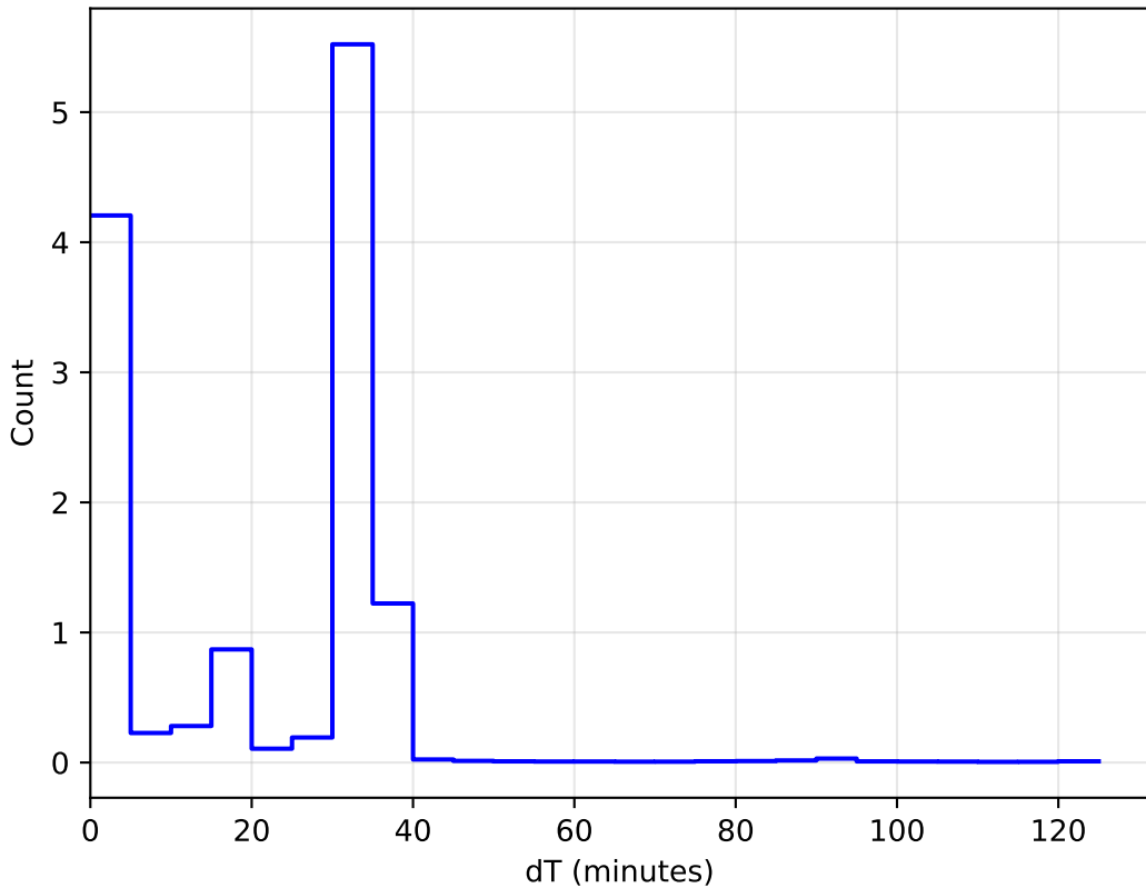
1e6 mw_roll_all_v3.3_10yrs All sky: DeltaT Histogram
