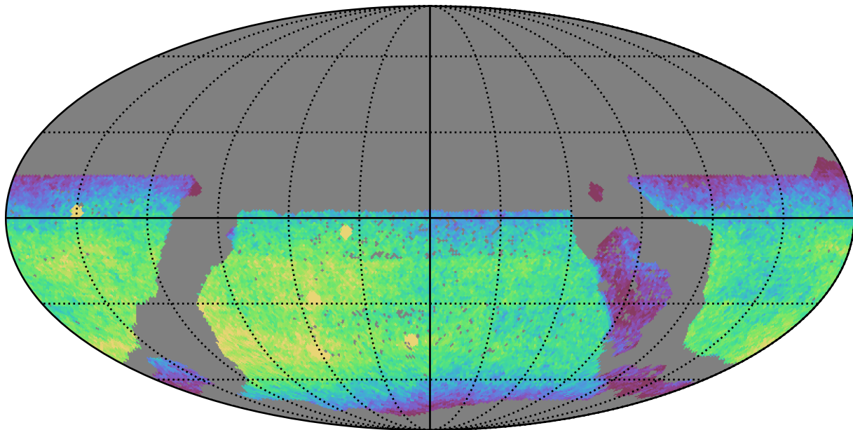
mw_roll_all_v3.3_10yrs WFD y band: CoaddM5
