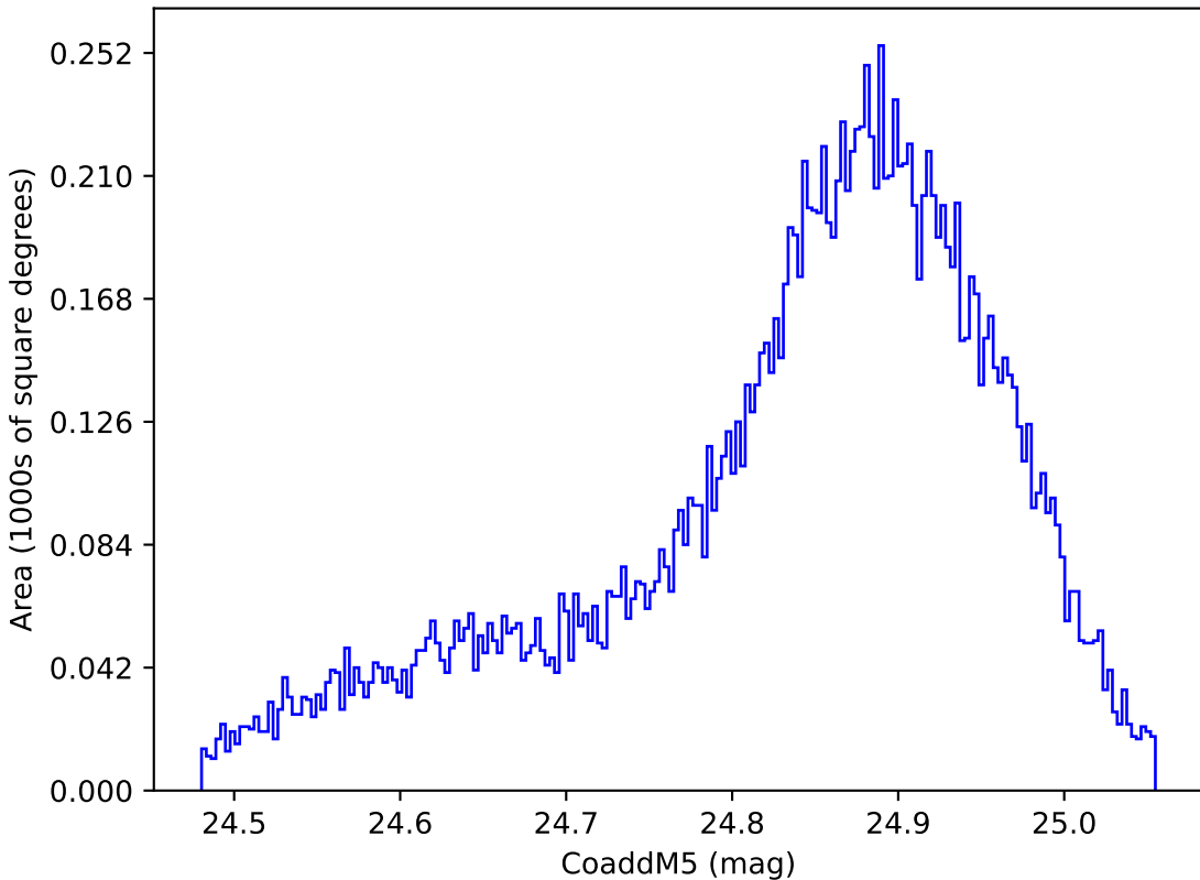
mw_roll_all_v3.3_10yrs WFD y band: CoaddM5
