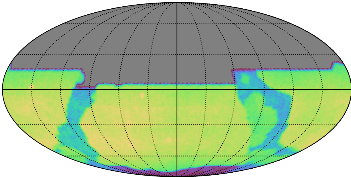
mw_roll_all_v3.3_10yrs All sky y band: CoaddM5
