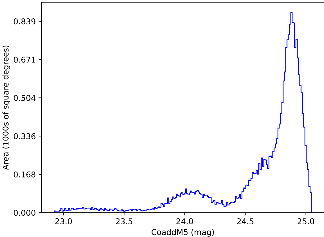
mw_roll_all_v3.3_10yrs All sky y band: CoaddM5
