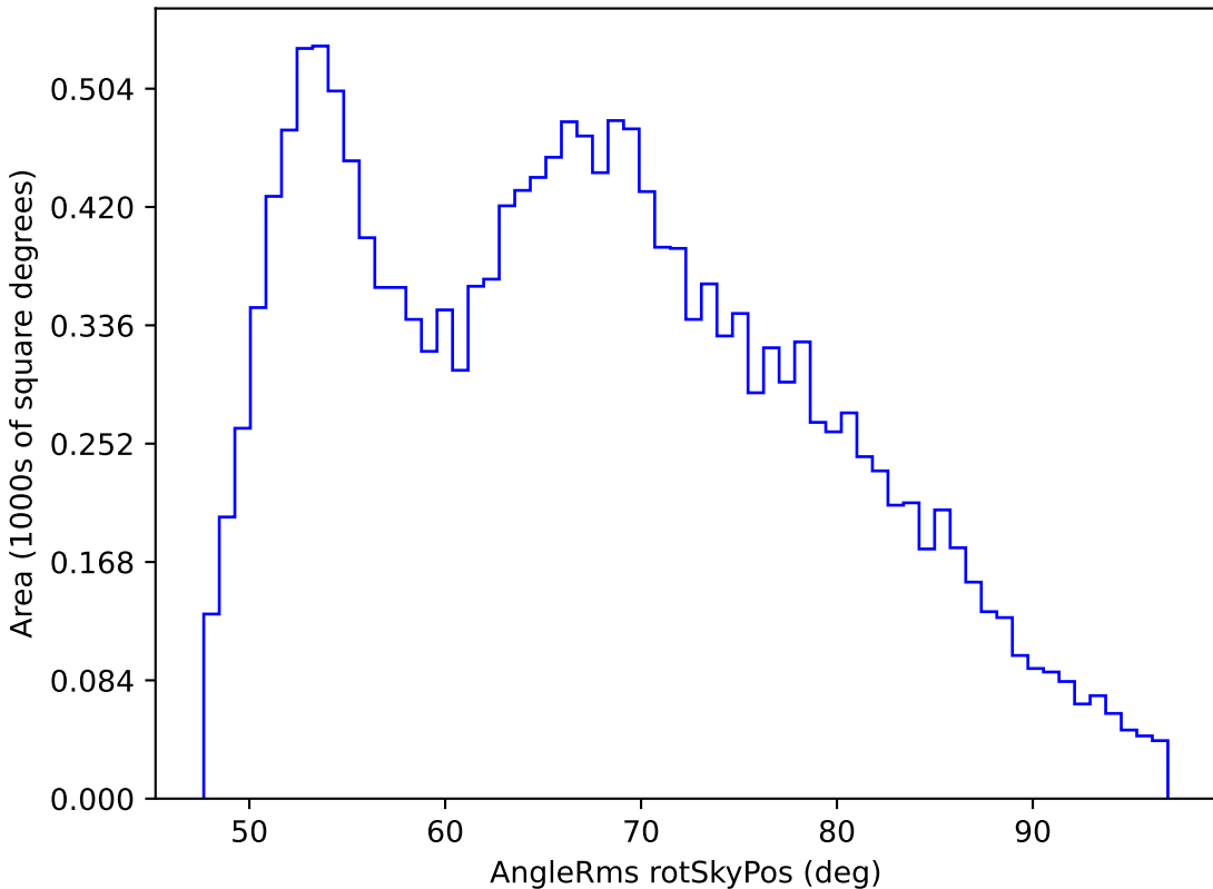
mw_roll_all_v3.3_10yrs WFD z band: AngleRms rotSkyPos
