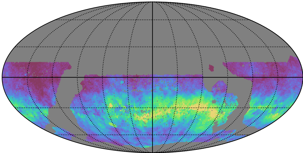
mw_roll_all_v3.3_10yrs WFD y band: AngleRms rotSkyPos
