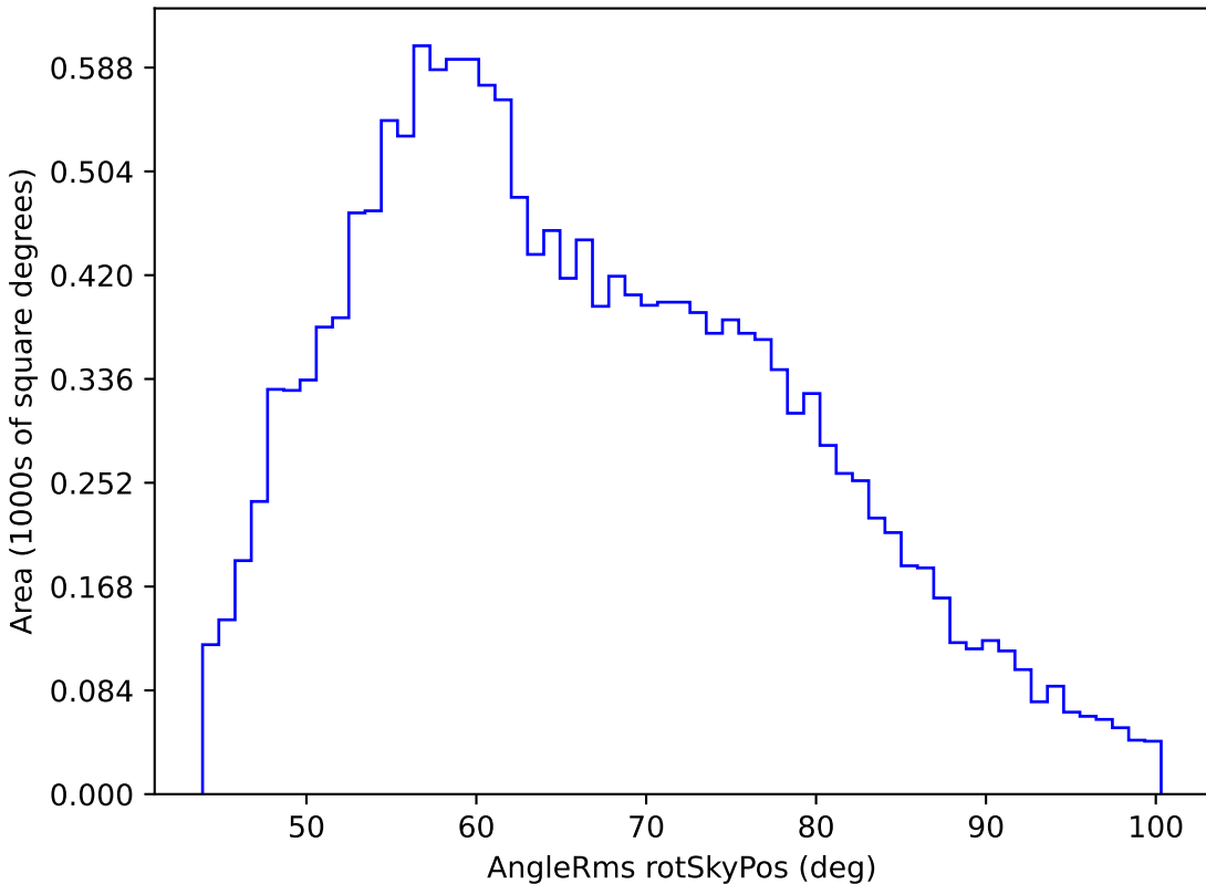
mw_roll_all_v3.3_10yrs WFD u band: AngleRms rotSkyPos
