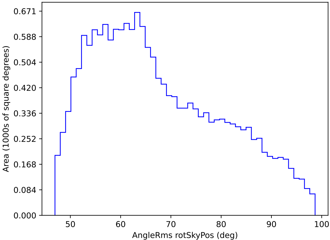
mw_roll_all_v3.3_10yrs WFD r band: AngleRms rotSkyPos
