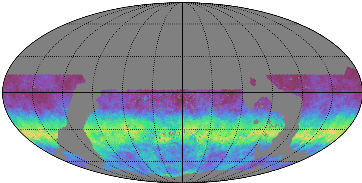
mw_roll_all_v3.3_10yrs WFD g band: AngleRms rotSkyPos
