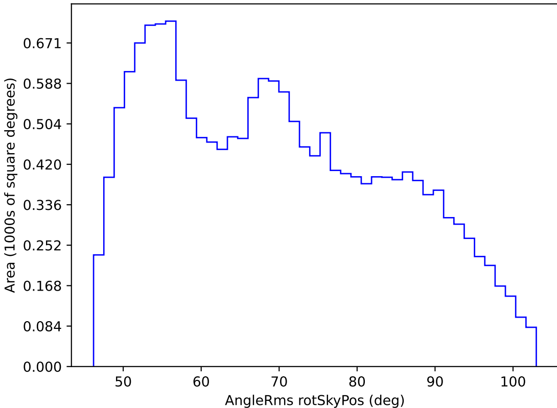
mw_roll_all_v3.3_10yrs WFD g band: AngleRms rotSkyPos
