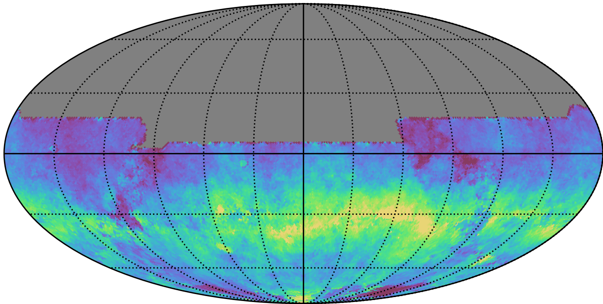
mw_roll_all_v3.3_10yrs All sky y band: AngleRms rotSkyPos
