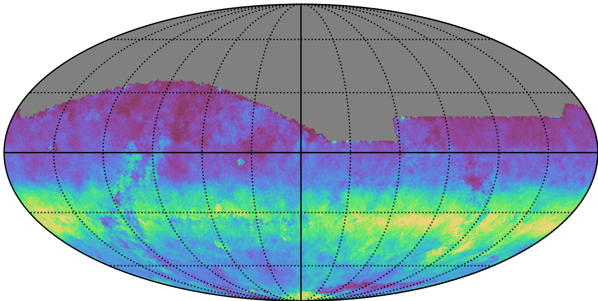
mw_roll_all_v3.3_10yrs All sky i band: AngleRms rotSkyPos
