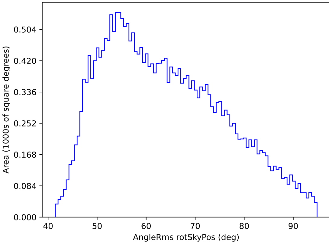
mw_roll_all_v3.3_10yrs All sky i band: AngleRms rotSkyPos
