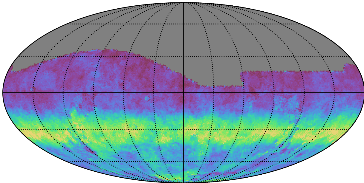
mw_roll_all_v3.3_10yrs All sky g band: AngleRms rotSkyPos
