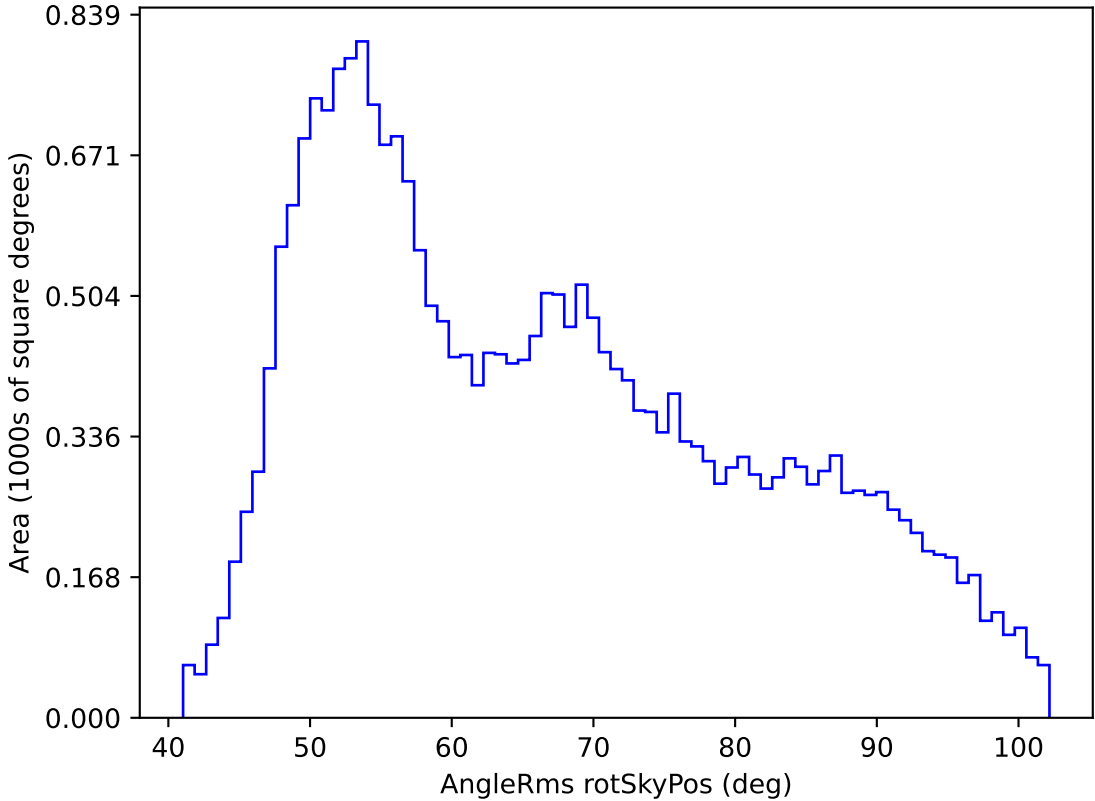
mw_roll_all_v3.3_10yrs All sky g band: AngleRms rotSkyPos
