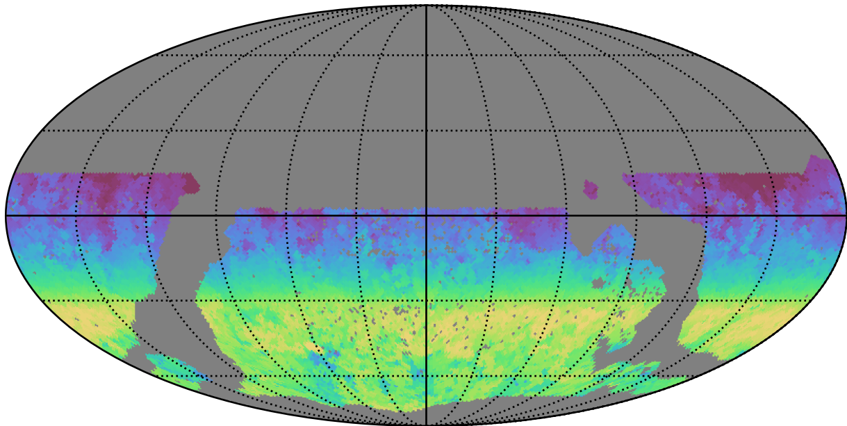
mw_roll_all_v3.3_10yrs WFD z band: AngleRange rotSkyPos
