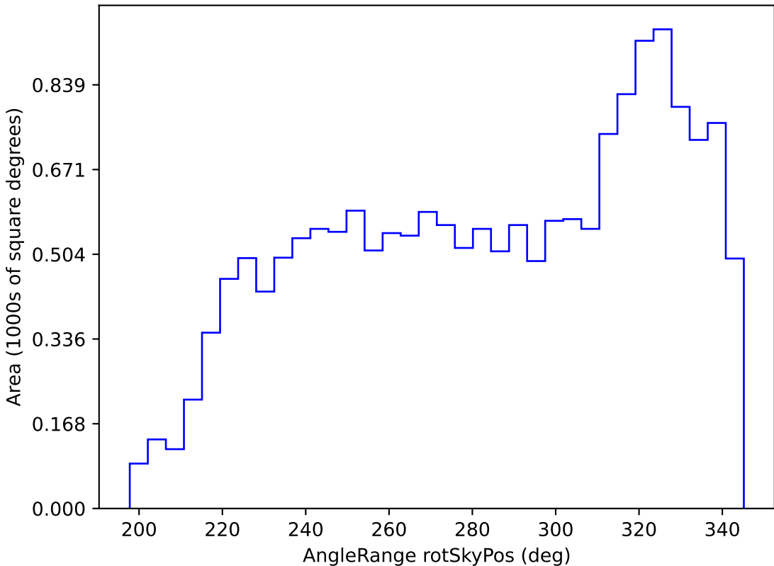
mw_roll_all_v3.3_10yrs WFD z band: AngleRange rotSkyPos
