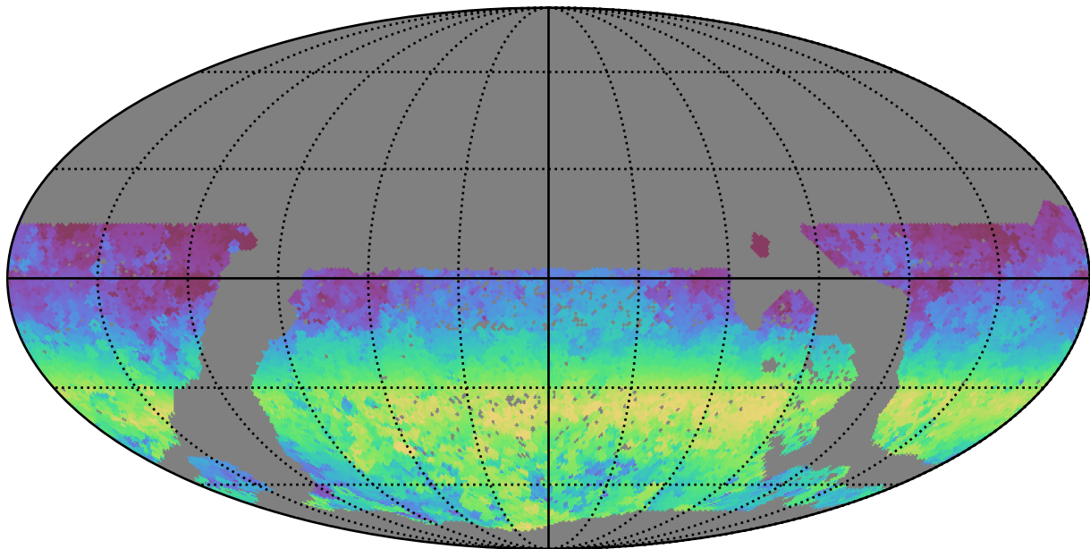
mw_roll_all_v3.3_10yrs WFD y band: AngleRange rotSkyPos
