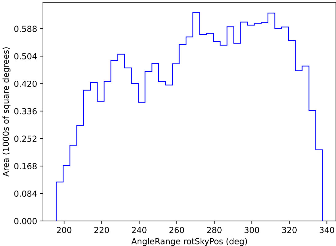
mw_roll_all_v3.3_10yrs WFD y band: AngleRange rotSkyPos
