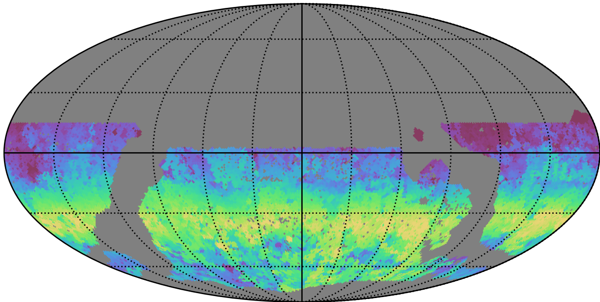
mw_roll_all_v3.3_10yrs WFD u band: AngleRange rotSkyPos
