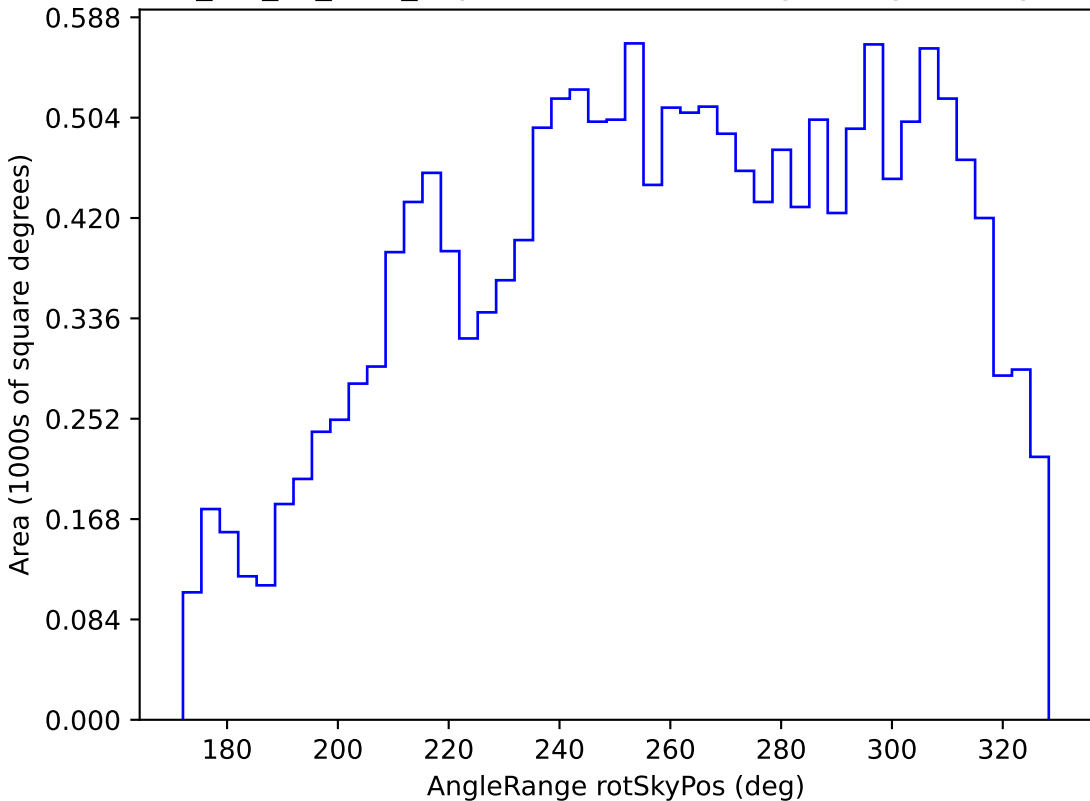
mw_roll_all_v3.3_10yrs WFD u band: AngleRange rotSkyPos
