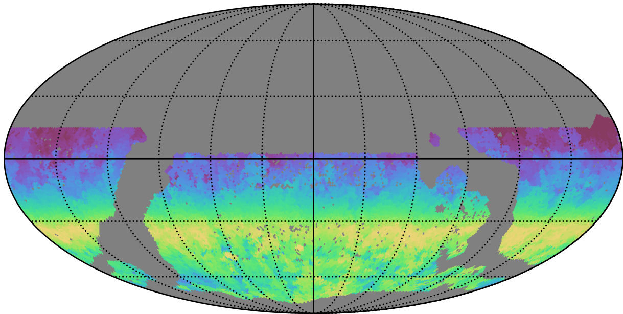
mw_roll_all_v3.3_10yrs WFD r band: AngleRange rotSkyPos
