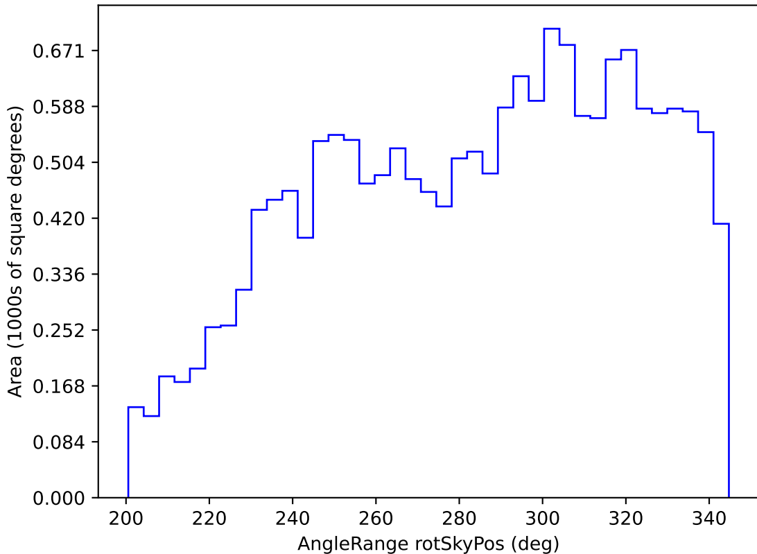
mw_roll_all_v3.3_10yrs WFD r band: AngleRange rotSkyPos
