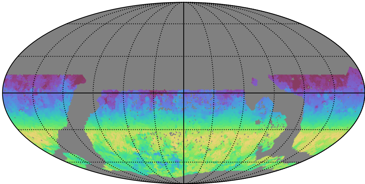
mw_roll_all_v3.3_10yrs WFD i band: AngleRange rotSkyPos
