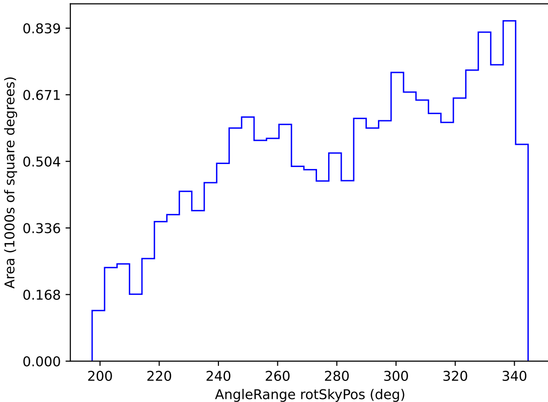
mw_roll_all_v3.3_10yrs WFD i band: AngleRange rotSkyPos
