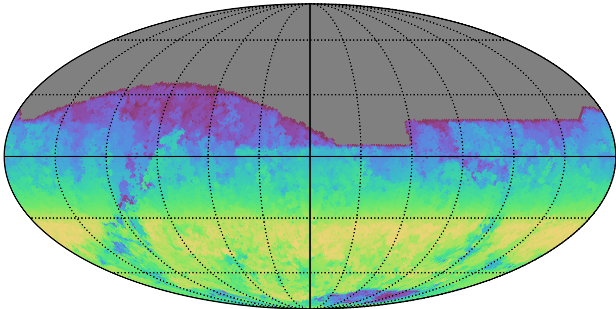
mw_roll_all_v3.3_10yrs All sky z band: AngleRange rotSkyPos
