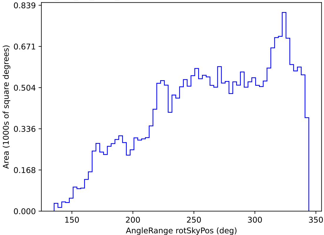
mw_roll_all_v3.3_10yrs All sky z band: AngleRange rotSkyPos
