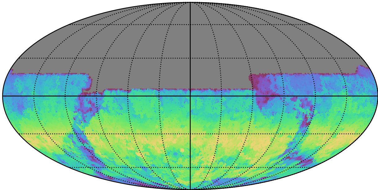
mw_roll_all_v3.3_10yrs All sky u band: AngleRange rotSkyPos
