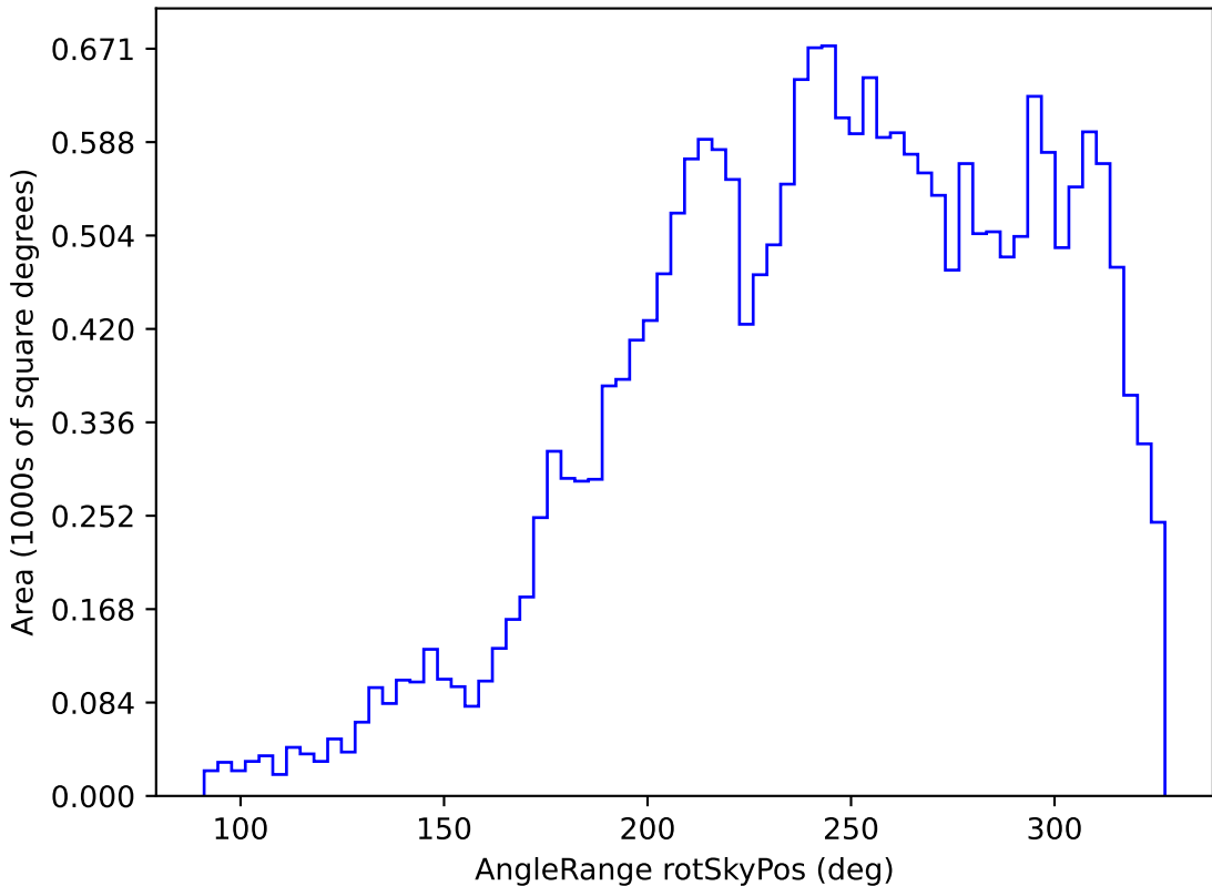
mw_roll_all_v3.3_10yrs All sky u band: AngleRange rotSkyPos
