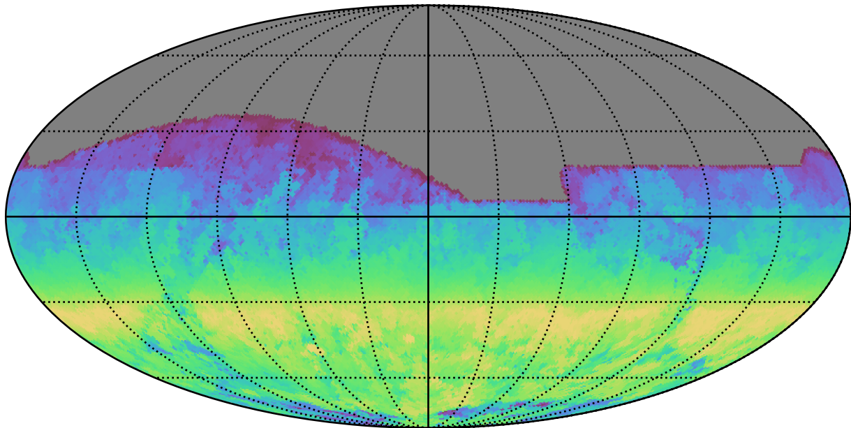
mw_roll_all_v3.3_10yrs All sky r band: AngleRange rotSkyPos
