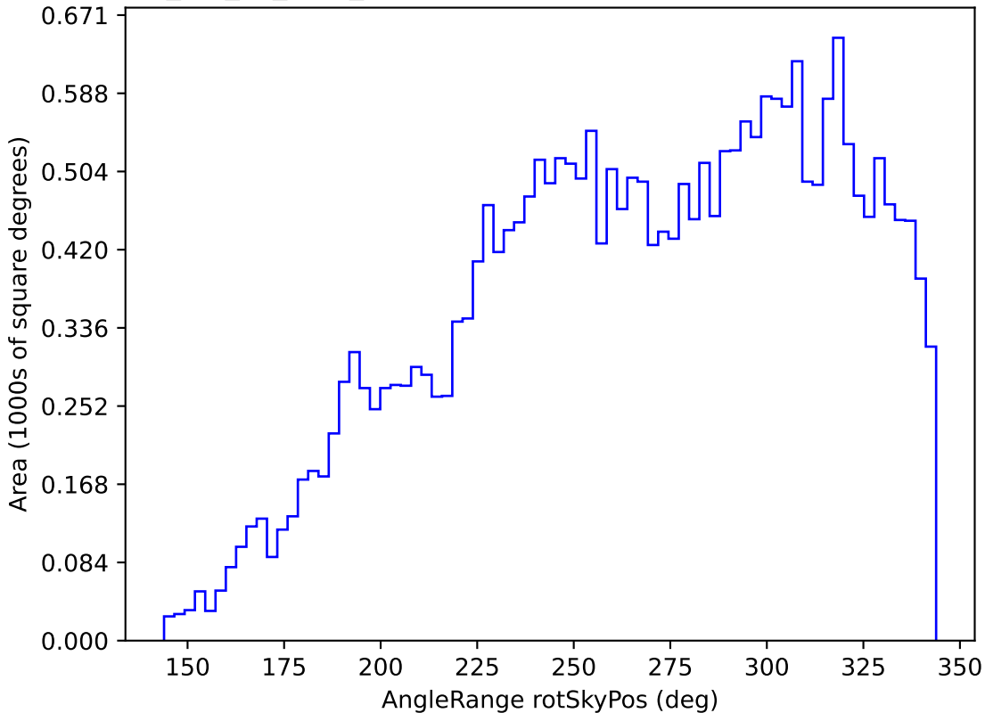
mw_roll_all_v3.3_10yrs All sky r band: AngleRange rotSkyPos
