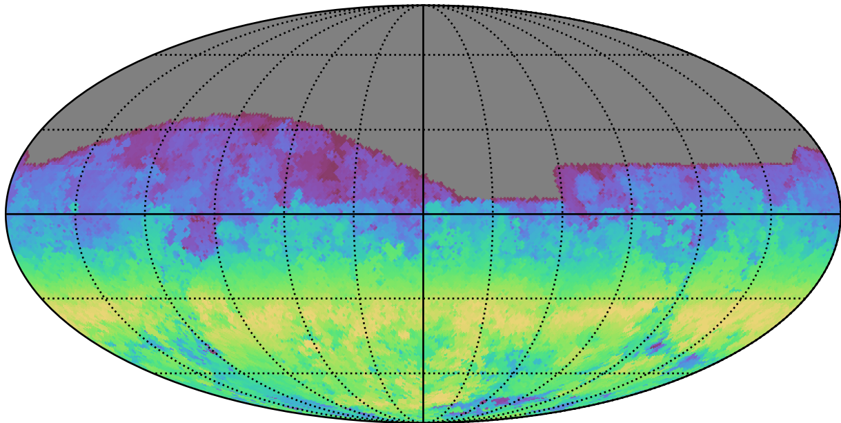
mw_roll_all_v3.3_10yrs All sky g band: AngleRange rotSkyPos
